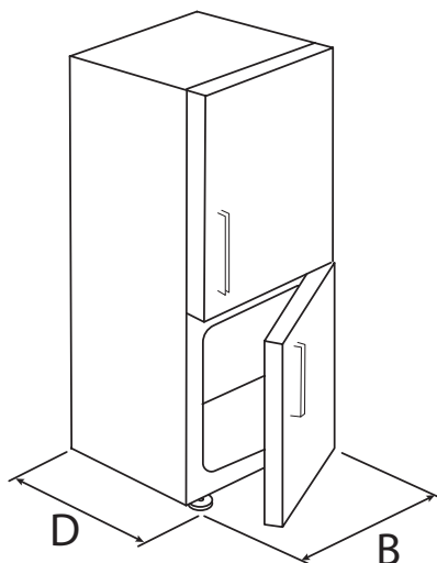
D mått mäts framkant fot (utan dörr)
